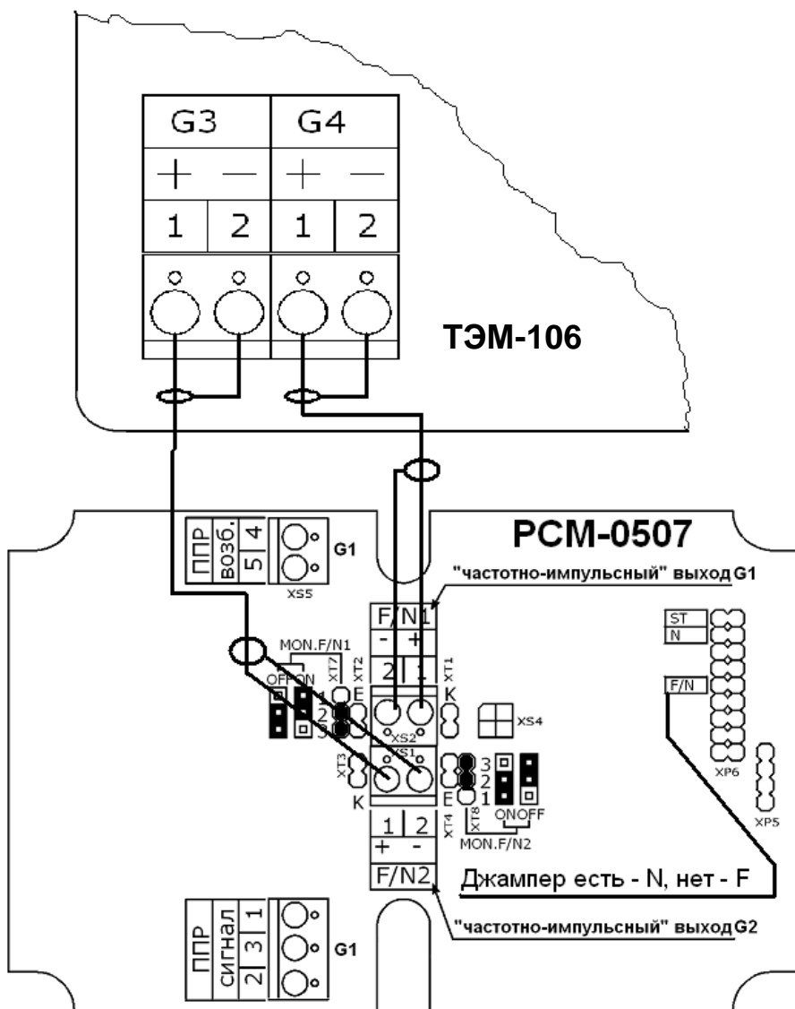
Рис. В.3в Подключение PCM-05.07
